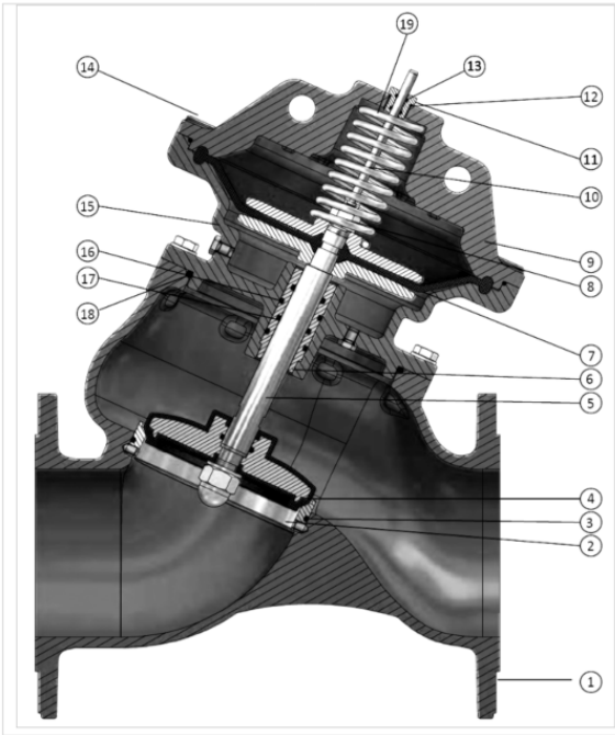
Устройство главной арматуры
